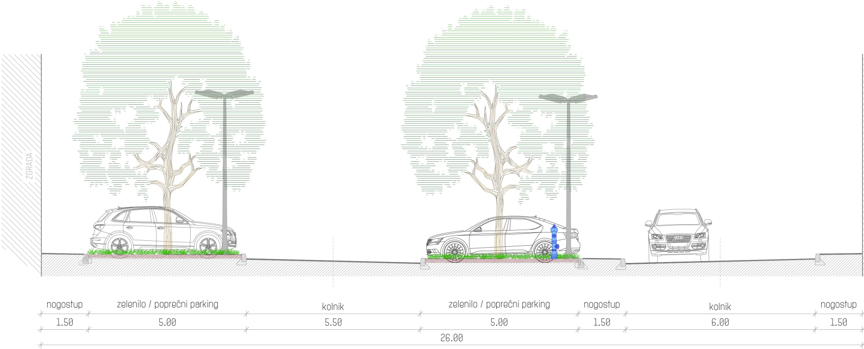
POPREČNI PRESJEK 1A
