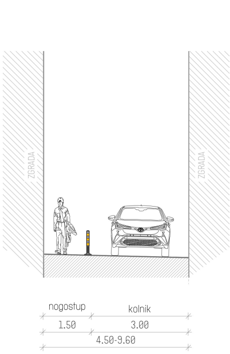
POPREČNI PRESJEK 3
