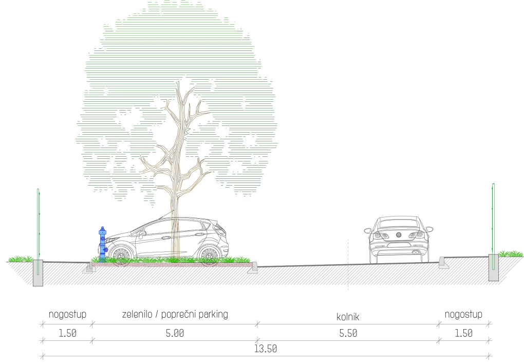
POPREČNI PRESJEK 1C
