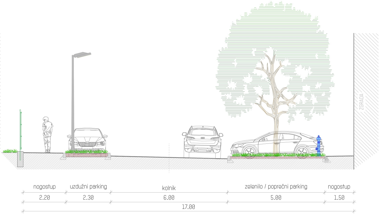
POPREČNI PRESJEK 1B
