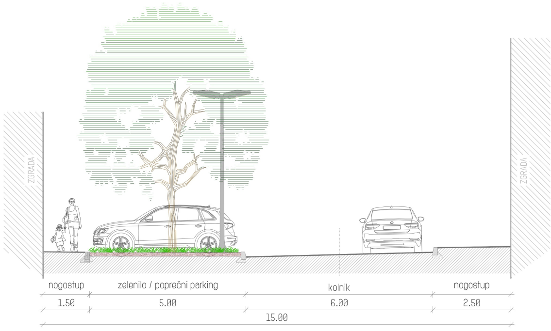
POPREČNI PRESJEK 2
