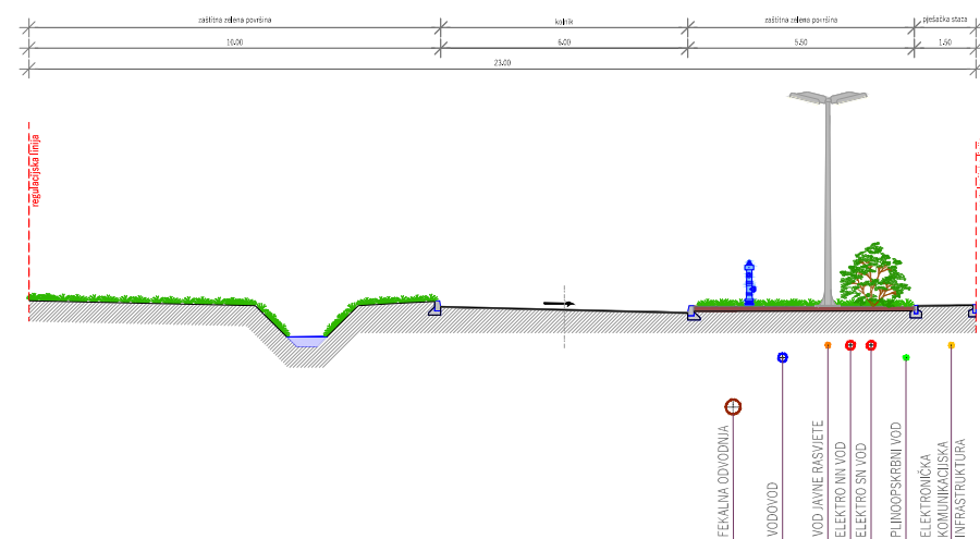
PRESJEK 3-3
